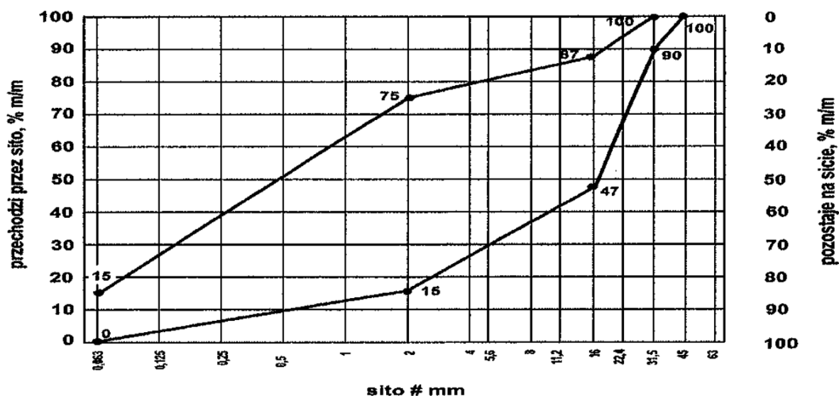
Rys. 1. Uziarnienie mieszanki kruszywa 0/31,5 do nawierzchni niezwiązanej.
